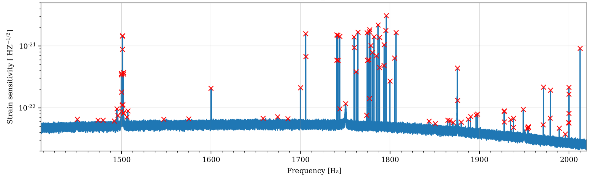
V1:Hrec_hoft_16384Hz
