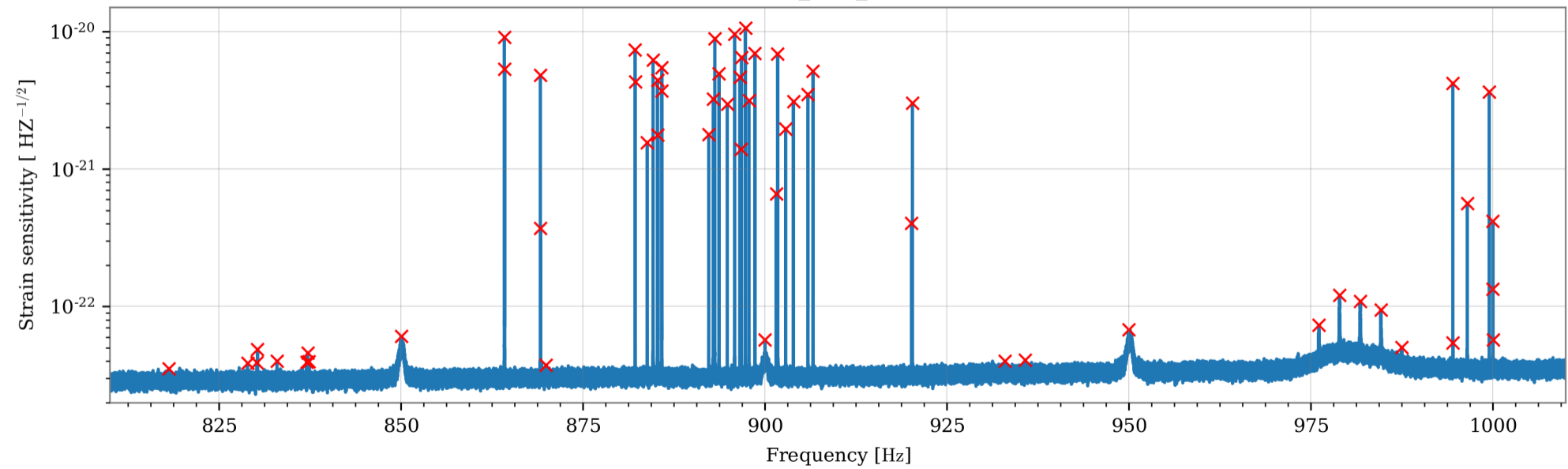
V1:Hrec_hoft_16384Hz
