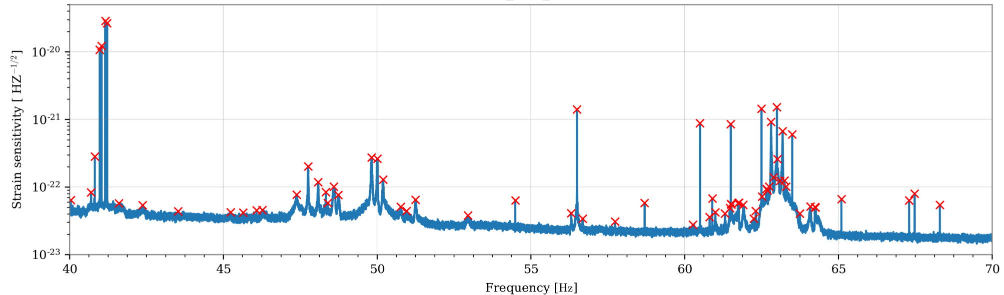
V1:Hrec_hoft_16384Hz
