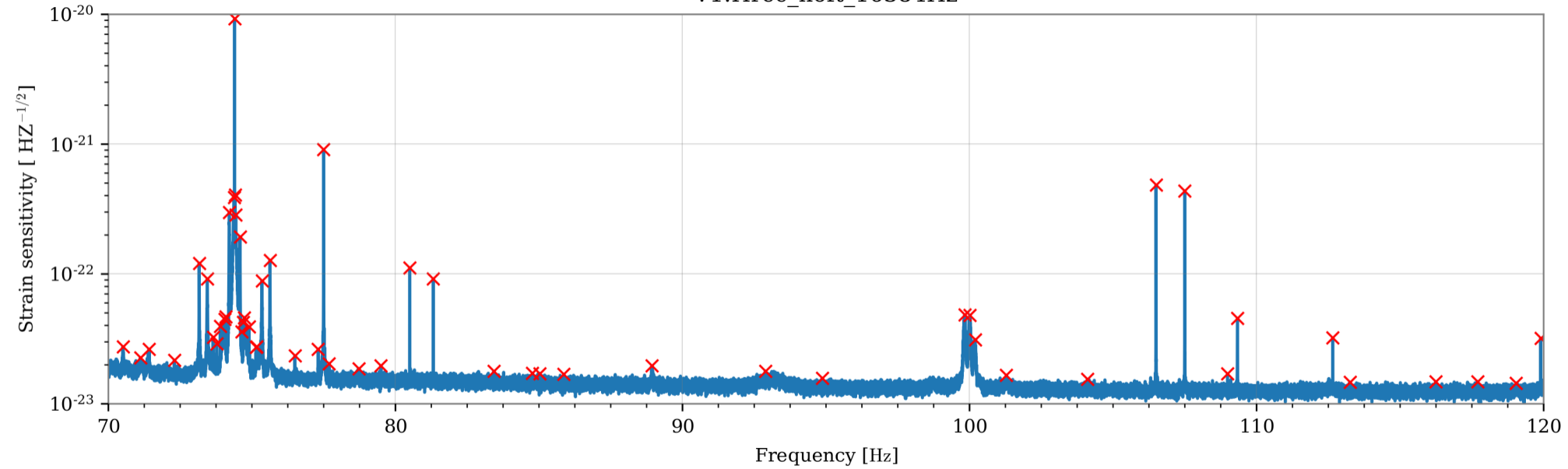
V1:Hrec_hoft_16384Hz
