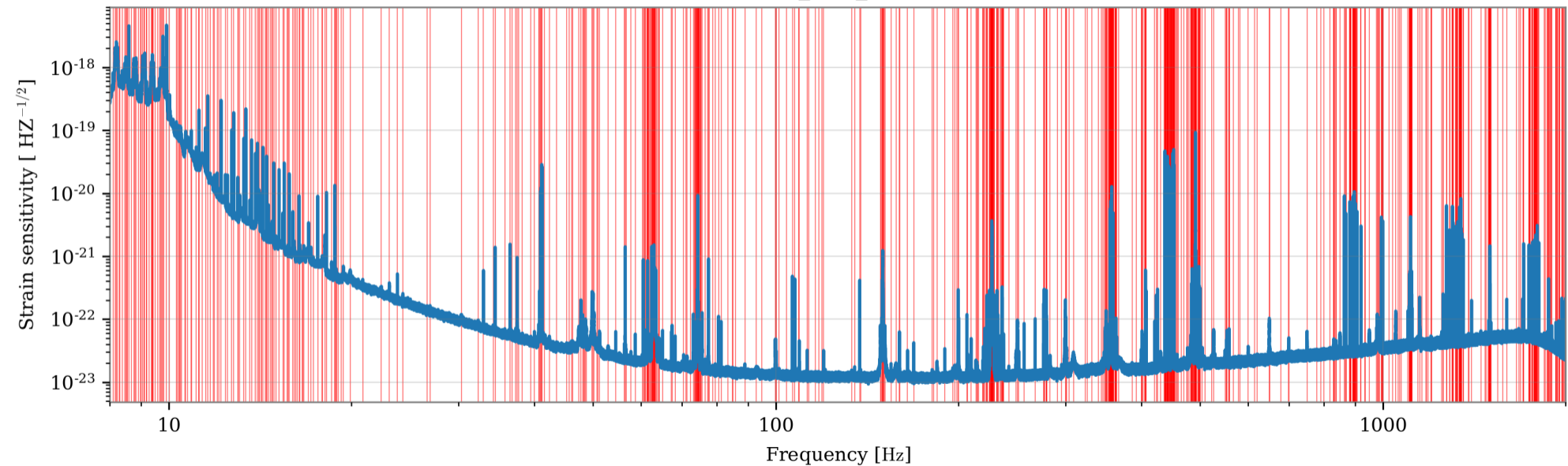
V1:Hrec_hoft_16384Hz
