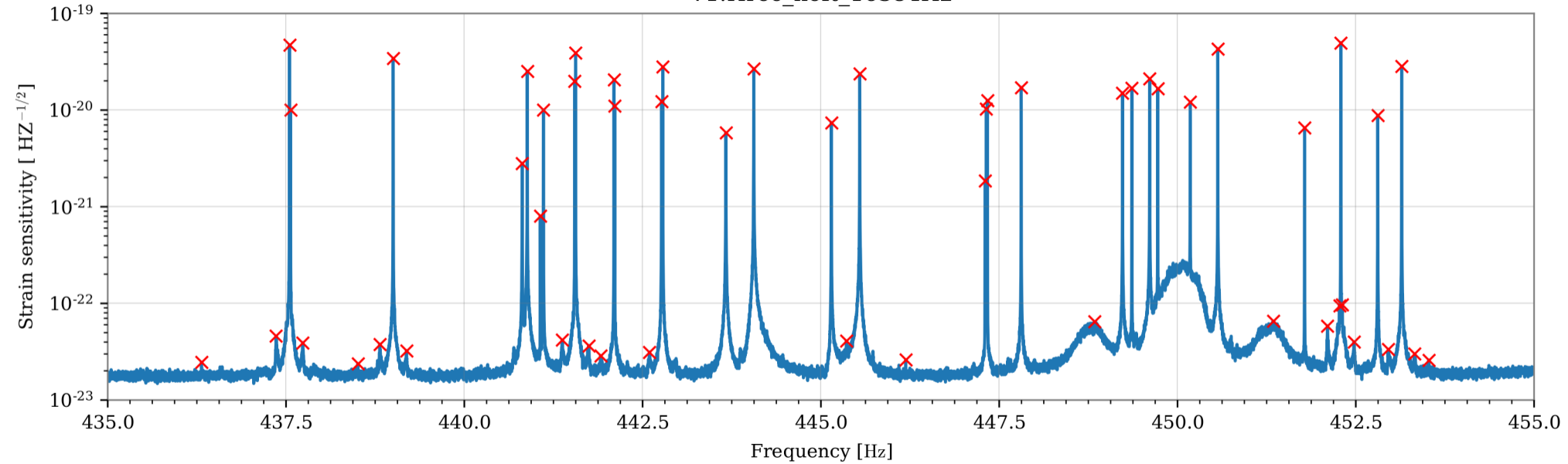
V1:Hrec_hoft_16384Hz
