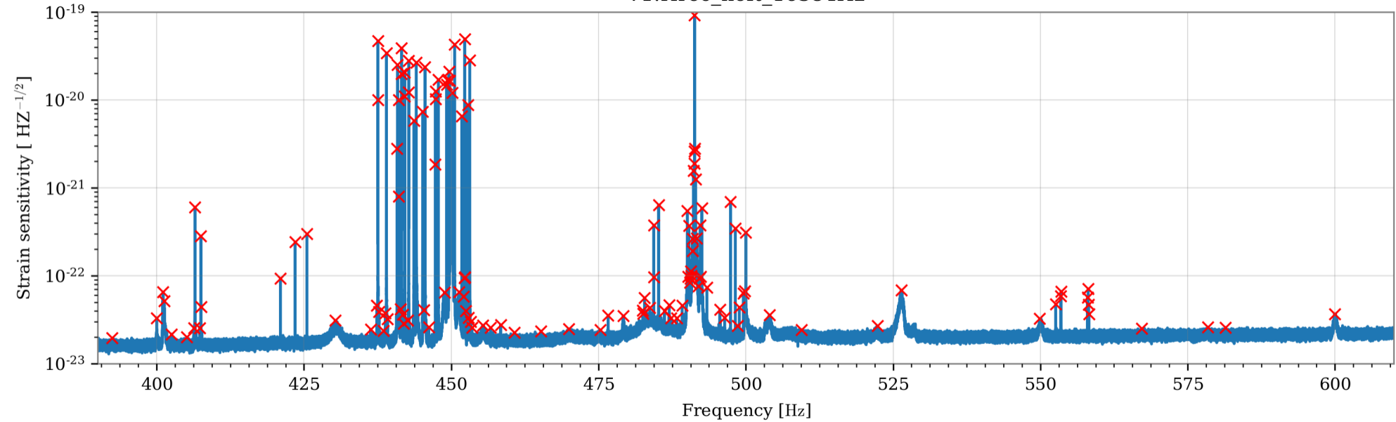
V1:Hrec_hoft_16384Hz
