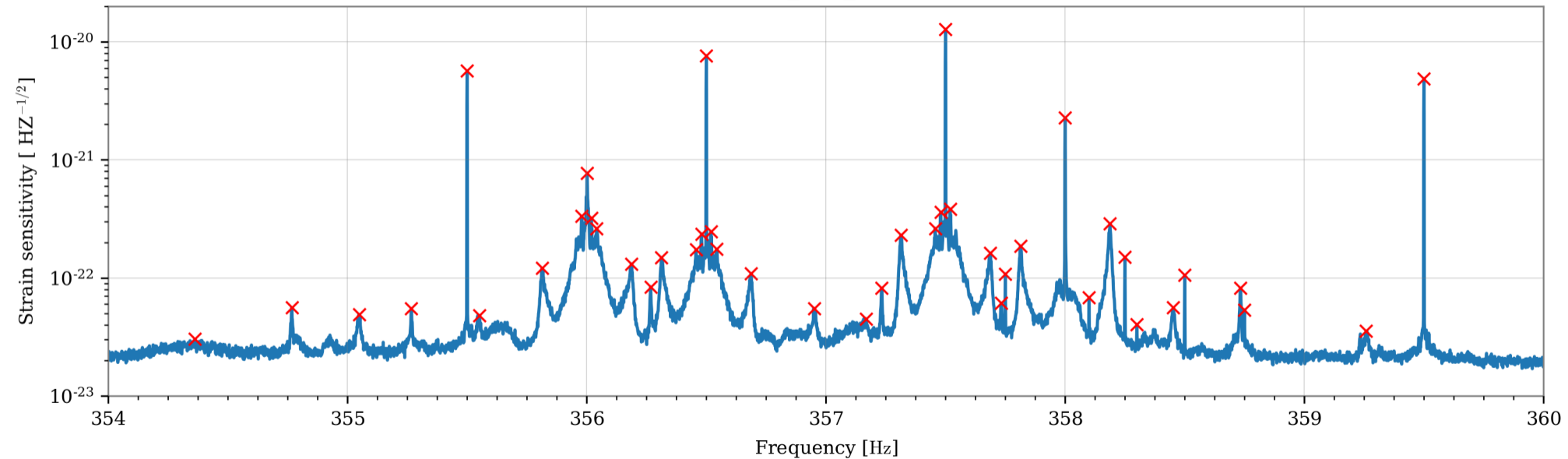
V1:Hrec_hoft_16384Hz
