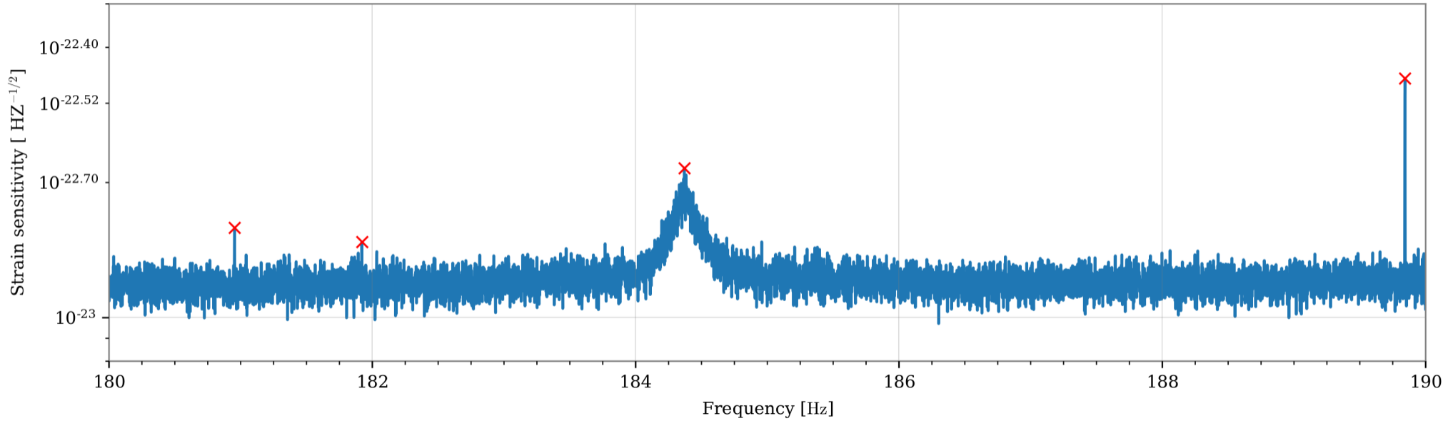
V1:Hrec_hoft_16384Hz
