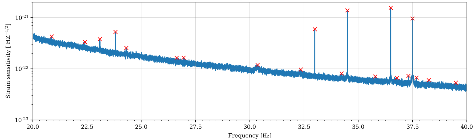
V1:Hrec_hoft_16384Hz
