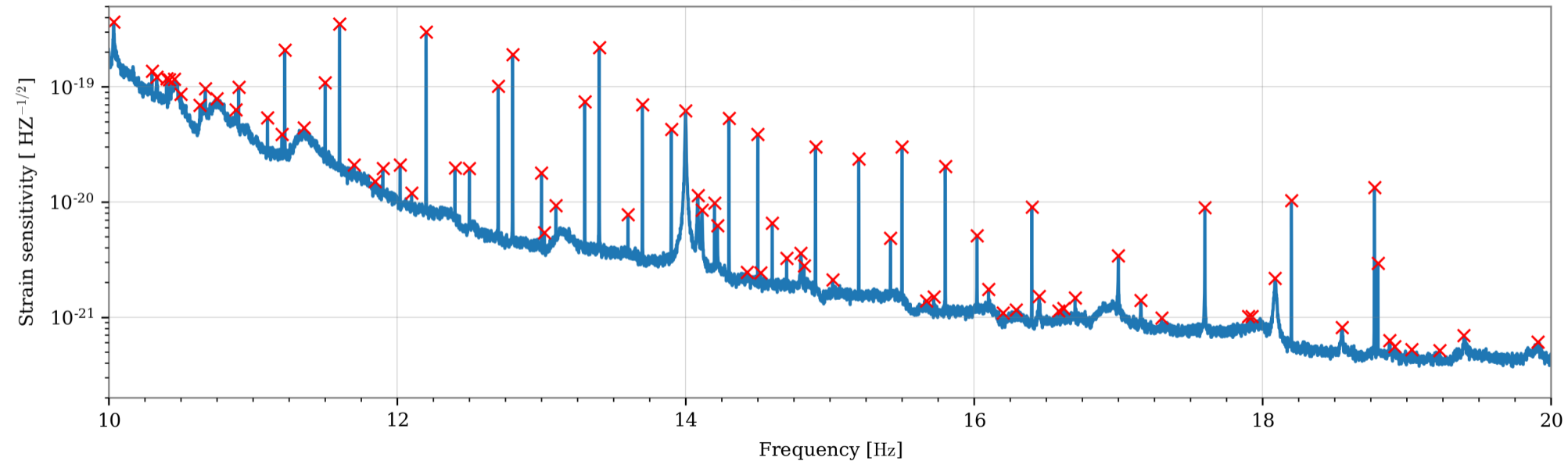
V1:Hrec_hoft_16384Hz
