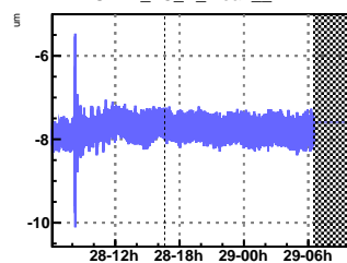
V1:SDB2_LC_Y_mean_TIME
