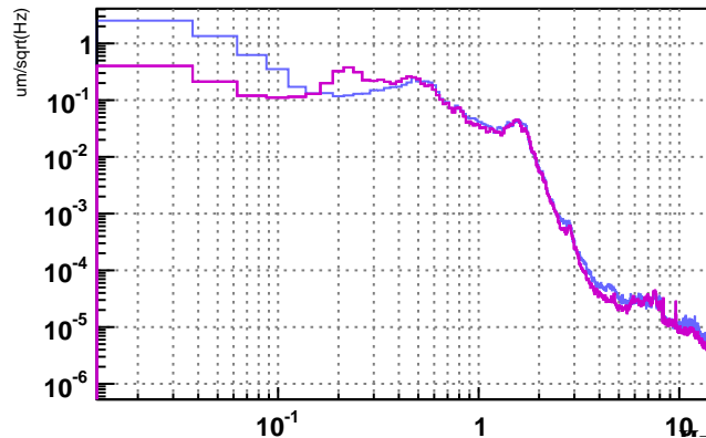
V1:SBE_SDB2_F0_z_500Hz__FFT
