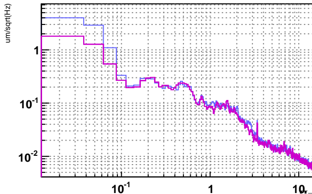
V1:Sa_OB_F0_Z_500Hz__FFT
