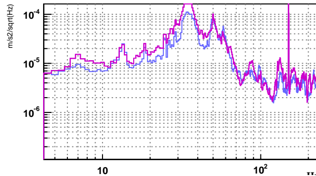
V1:ENV_SQZ_ACC_Y_FFT
