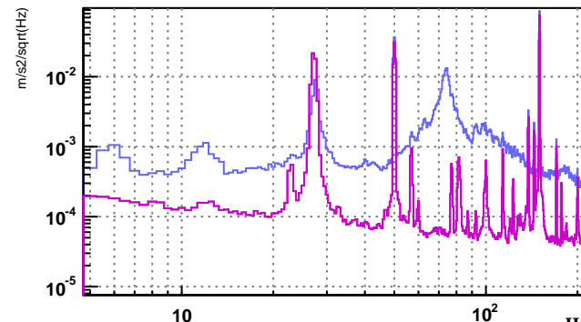
V1:ENV_SQZ_MINI_ACC_FFT
