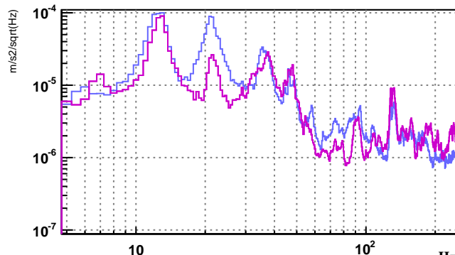
V1:ENV_SQZ_ACC_Z_FFT
