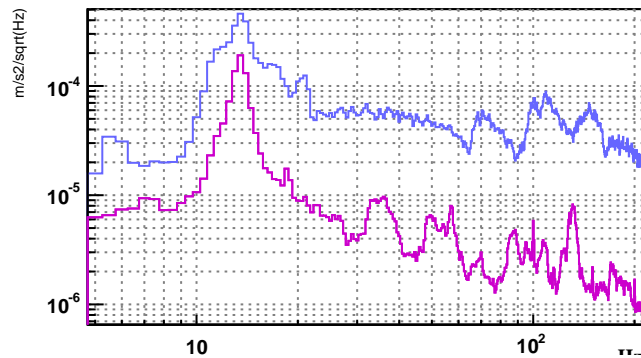
V1:ENV_SQZ_ACC_X_FFT
