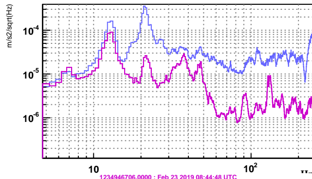
V1:ENV_SQZ_ACC_Z_FFT
