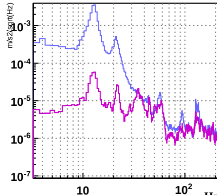
V1:ENV_SQZ_ACC_Z_FFT
