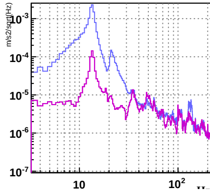
V1:ENV_SQZ_ACC_X_FFT
