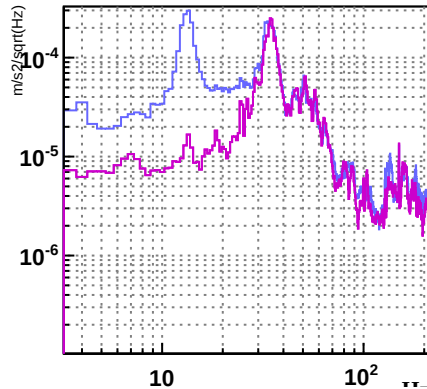
V1:ENV_SQZ_ACC_Y_FFT
